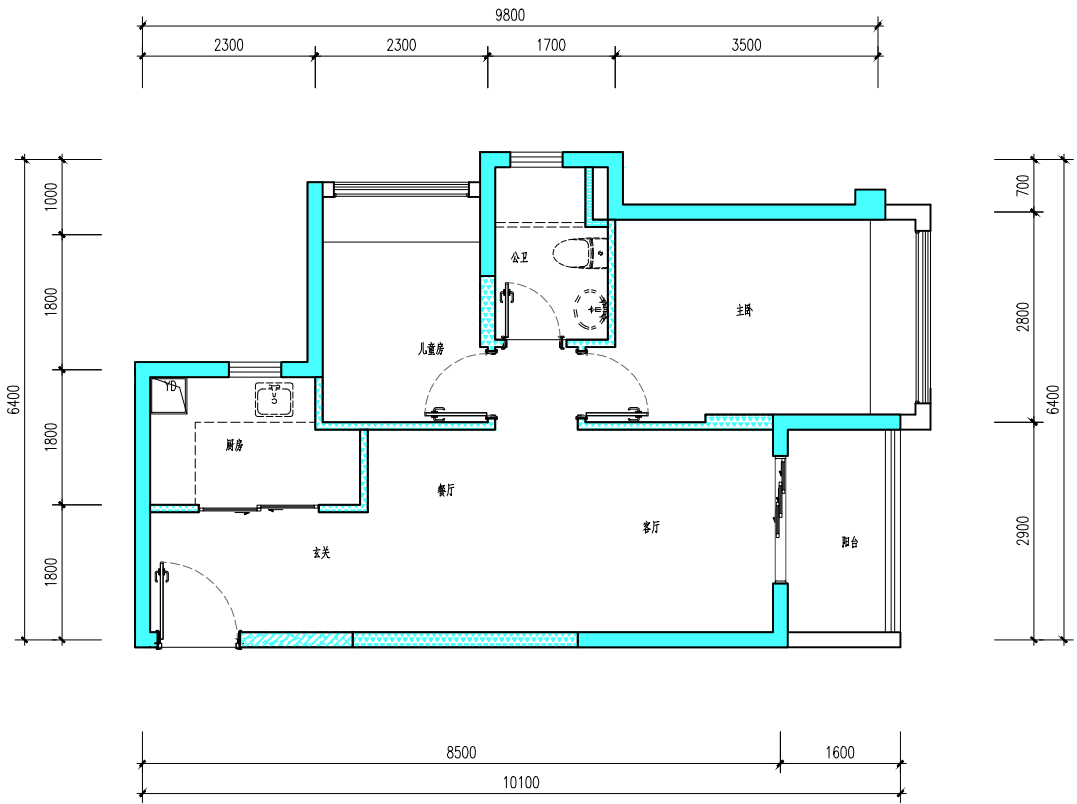
六单元02户型平面图
