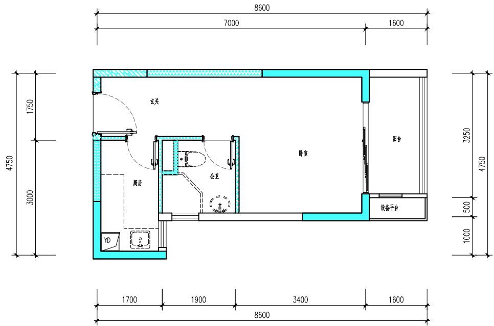
六单元03户型平面图
